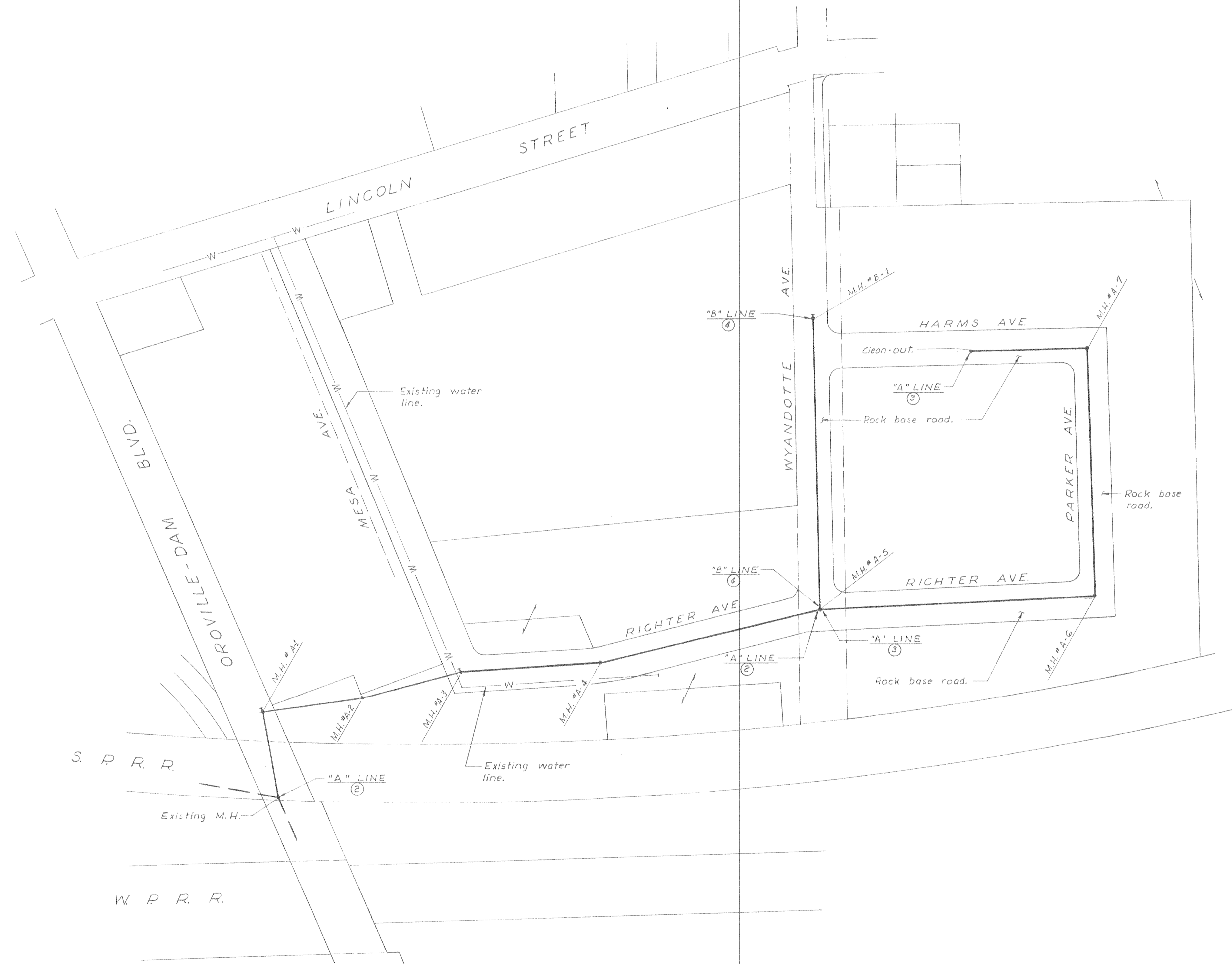
SEWER LAYOUT Scale: 1" = 100'
